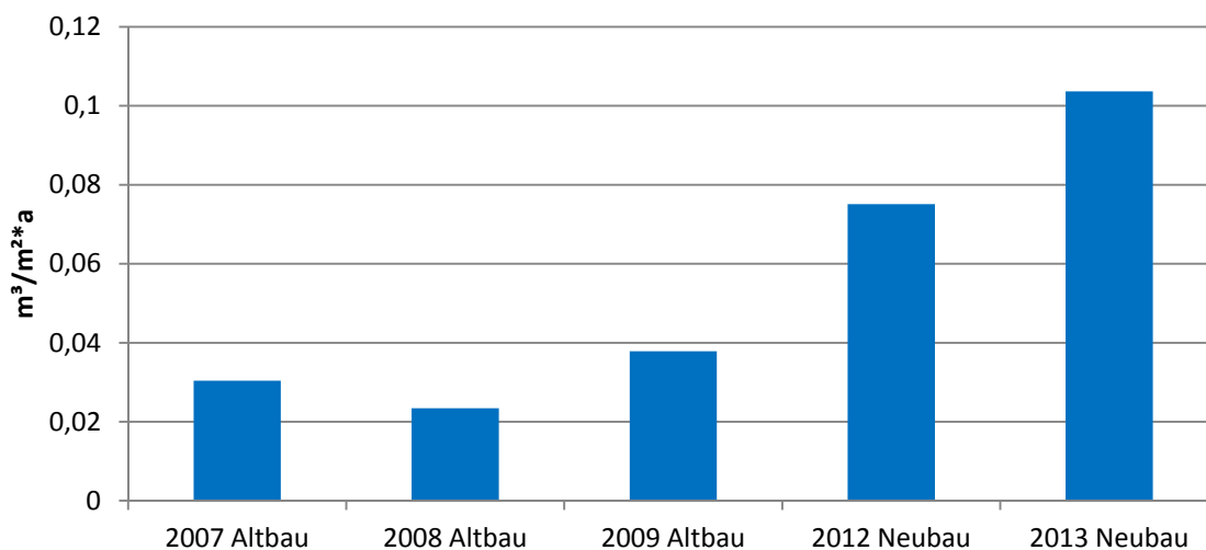
Abbildung 53: Jährlicher Wasserverbrauch Schillerschule auf Esch
