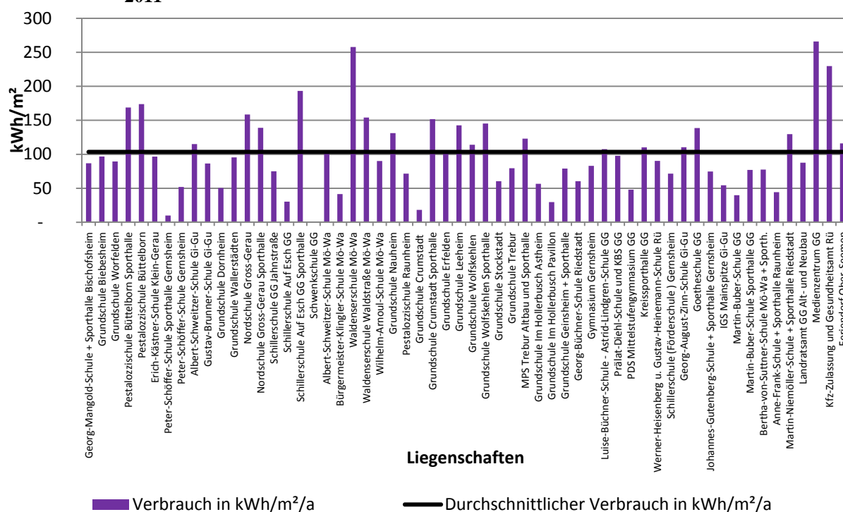
Abbildung 31: Spezifischer Heizenergieverbrauch witterungsbereinigt der Liegenschaften in kWh/m 2 2011
