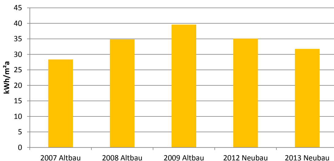
Abbildung 52: Jährlicher Stromverbrauch Schillerschule auf Esch
