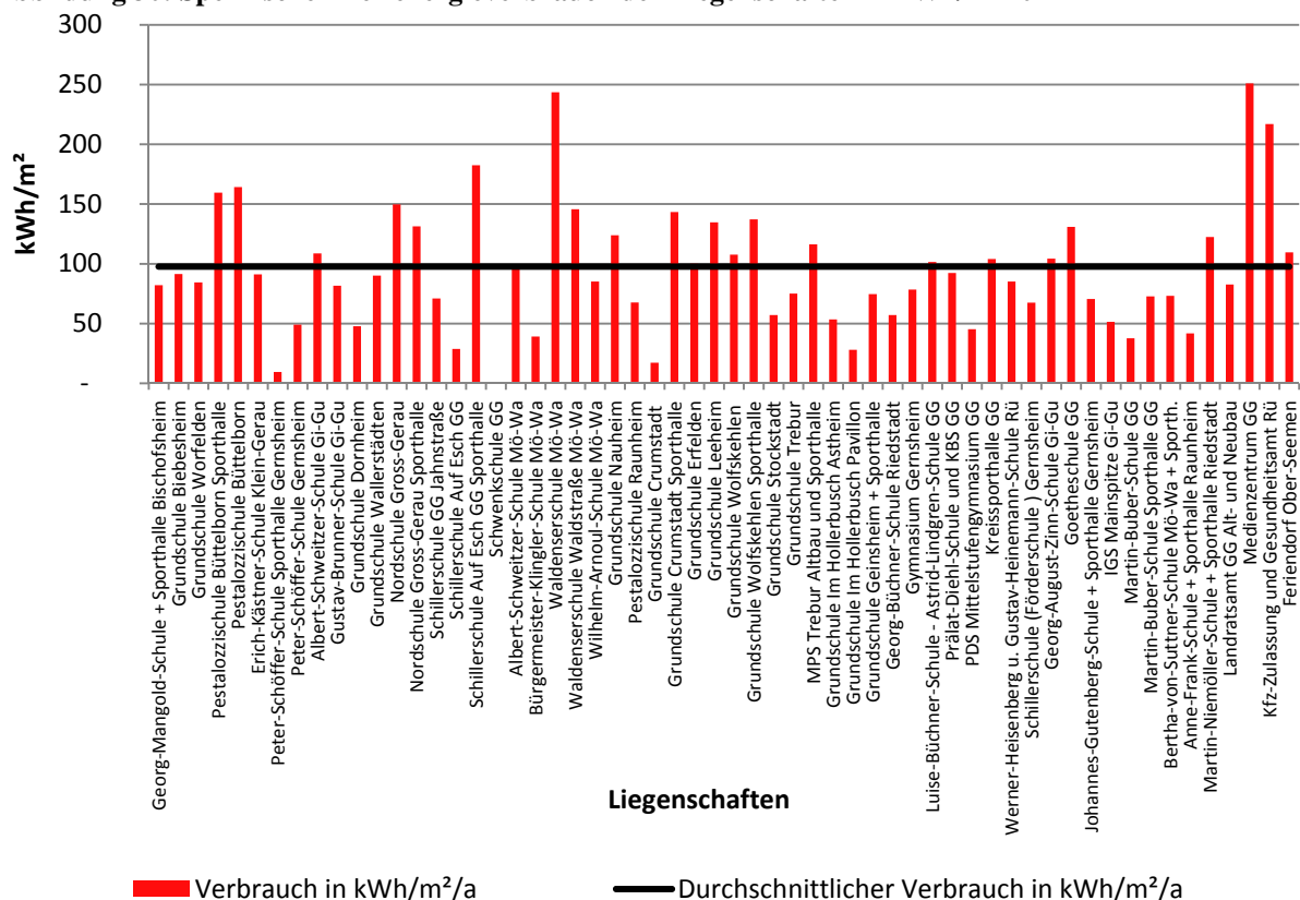
Abbildung 30: Spezifischer Heizenergieverbrauch der Liegenschaften in kWh/m 2 2012
