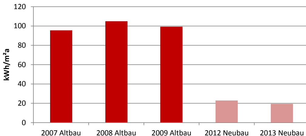
Abbildung 51: Jährlicher Endenergiebedarf Schillerschule auf Esch
