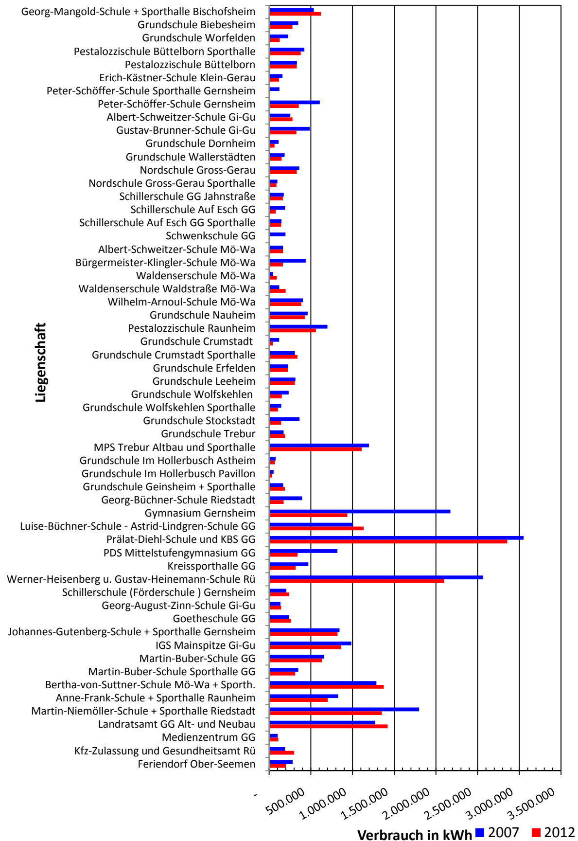
Abbildung 27: Witterungsbereinigter Heizenergieverbrauch im Vergleich zwischen den Jahren 2007 und 2012
